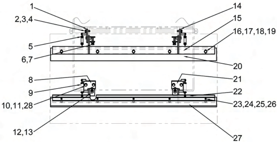
VIEW A-A
